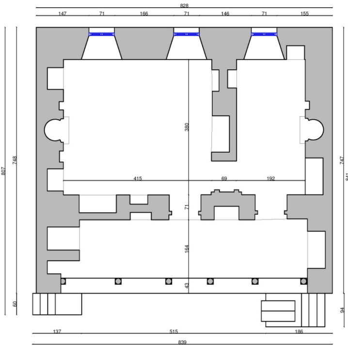
Дом М.Ф.Ахундова. План
