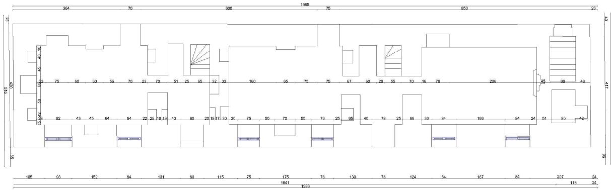
Дом Шекихановых. План 1-го и 2-го этажей
