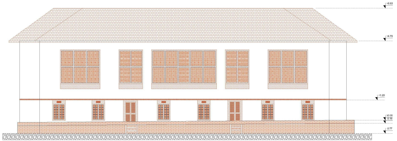
Дом Шекихановых. Фасад
