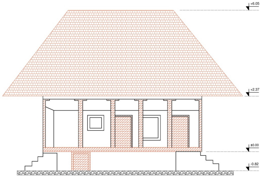
Дом М.Ф.Ахундова. Фасад
