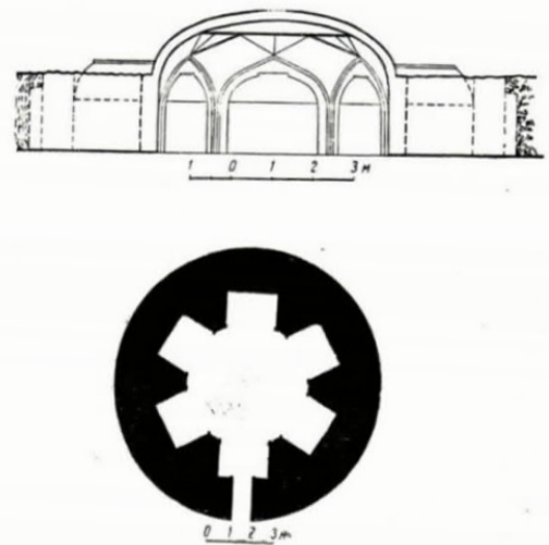
Рисунок 3. Мавзолей Ахсадан Баба. План и фасад.
